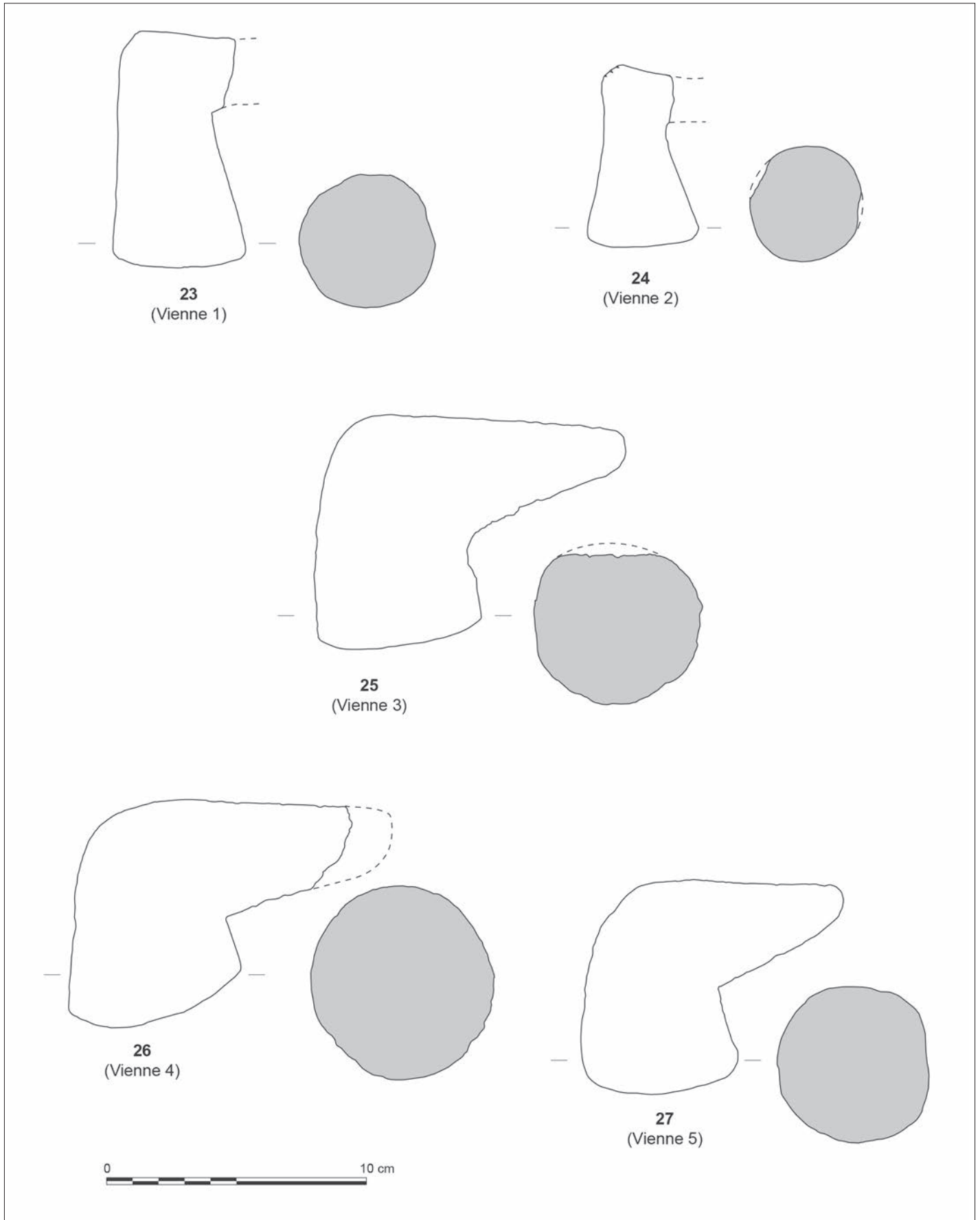
Fig. 20 – Broyeurs de Vienne (Isère) (dessin : Y. Manniez ; DAO : V. Lauras).
