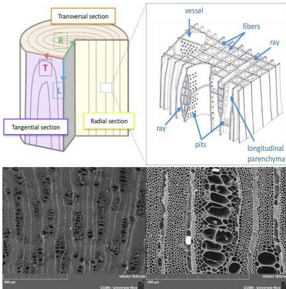
Fig.3 : En haut : schéma tridimensionnel de la structure anatomique d'un bois d'angiosperme (d'après Trouy, 2015). En bas : image au microscope électronique à balayage d'une coupe transversale d'un charbon archéologique de Boscia sp.
