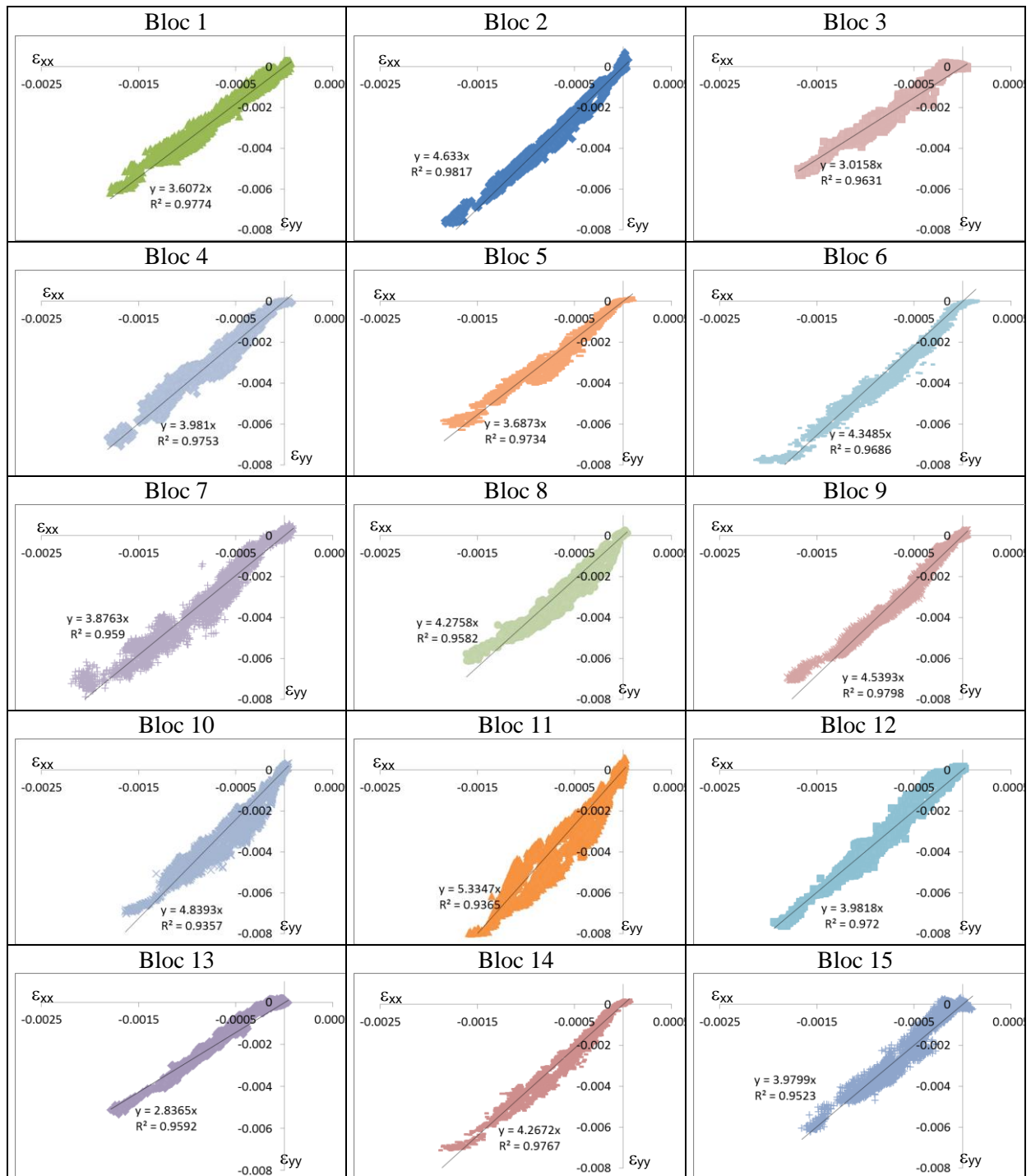
Figure 4. Evolution des déformations \epsilon_{yy} par rapport aux déformations \epsilon_{xx} pour les quinze blocs. Les valeurs des pentes affichées correspondent à 1/\Gamma .
