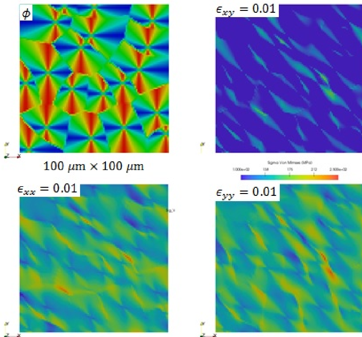
FIGURE 2 – (a) Champs d’orientation des cristallites \phi , (b) champ de contrainte équivalente de von Mises pour une déformation macroscopique de cisaillement avec des conitions aux limites périodiques et pour une élongation suivant x (c) puis suivant y (d).
