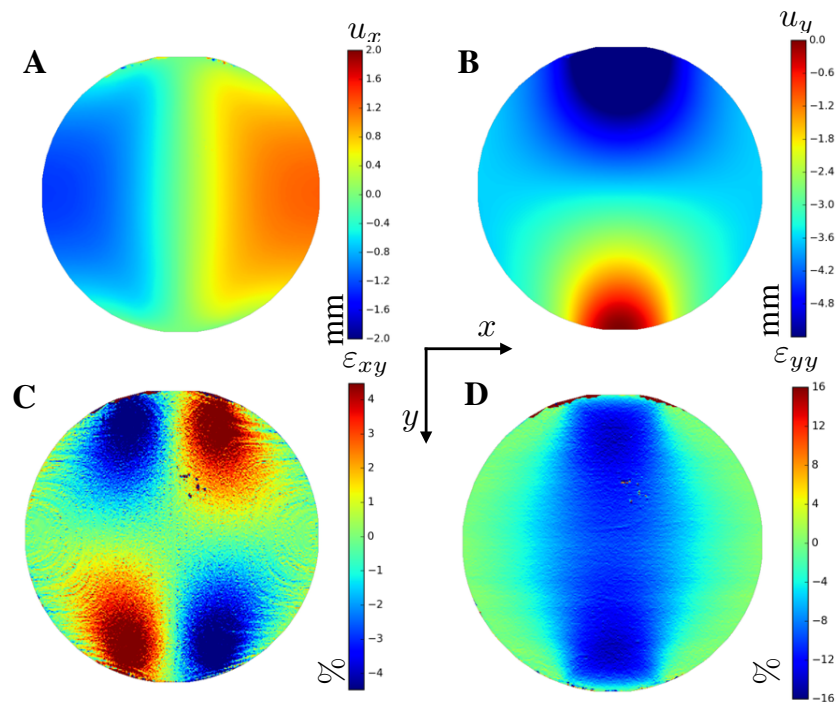
Figure 2: A,B: Le champ de déplacement mesuré par corrélation d'images selon les directions x et y . C,D: Champ de déformation de deux composantes \varepsilon_{xy} et \varepsilon_{yy} . Les champs sont tracés sur la géométrie non déformée pour une déformation globale de 14% de la particule. Les mesures sont bruitées à la frontière car les cellules de corrélation impliquant une zone hors du disque présentent un déficit d'information.
