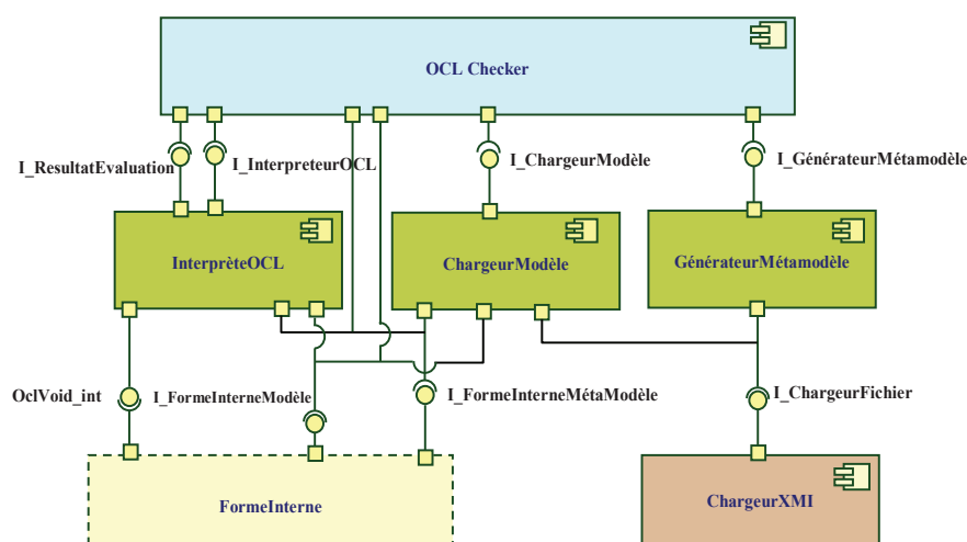
Figure 11. Architecture de la plate-forme NEPTUNE II
