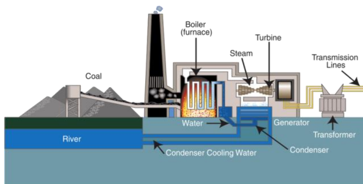
Process d'une centrale thermique à base d'input charbon
