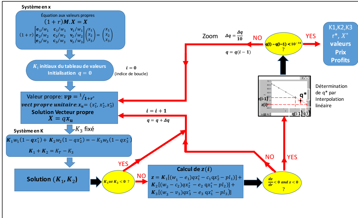
Figure 12. Schéma de l'algorithme dans le cas 3 branches avec capital fixe nul.
