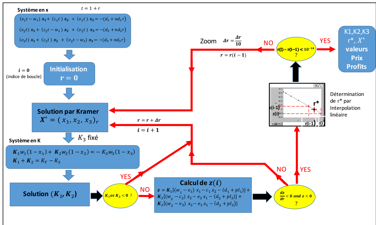
Figure 11. Schéma de l'algorithme dans le cas 3 branches avec capital fixe différent de zéro. La donnée du problème est un tableau de valeurs correspond à une répartition à priori arbitraire des capitaux mais fixant les coefficients socio-techniques.
