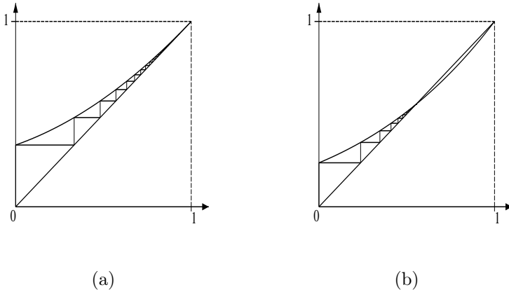
Рис. 9.2: Графік функцій y = f(x) та y = x . Ймовірність зникнення x_n = f(x_{n-1}) в межах n - це висота n -го «кроку сходів». (а): f(x) = (1 + x + x^2)/3 . (б): f(x) = (3 + x)^5/4^5 .
