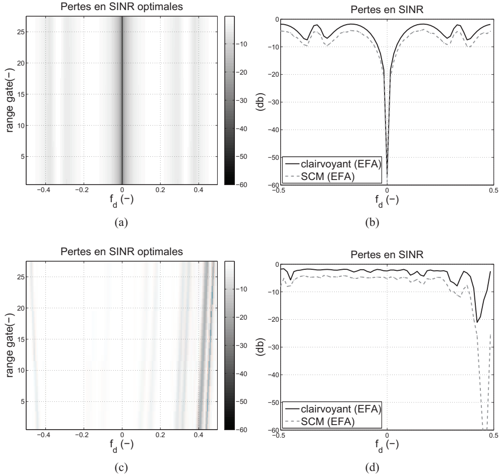
Figure 5. Non-stationnarité du fouillis. (a) Pertes en SINR optimal pour un radar en visée latérale \phi_a = 0 . (b) Pertes en SINR pour la case 14 pour un radar en visée latérale \phi_a = 0 . (c) Pertes en SINR optimal pour un radar en visée frontale \phi_a = -\pi/2 . (d) Pertes en SINR pour la case 14 pour un radar en visée frontale \phi_a = -\pi/2 .
