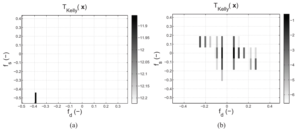
Figure 6. Statistique de test du détecteur de Kelly pour un cas multicibles. (a) Détection sur la pleine dimension NM . (b) Détection dans une structure EFA sur la dimension NM' \ll NM .
