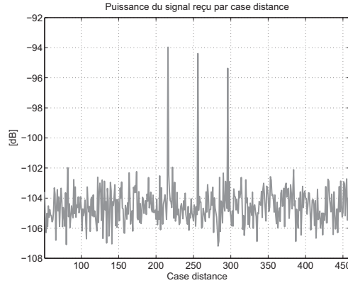
Figure 3. Puissance reçue pour une rafale en fonction de la distance.
