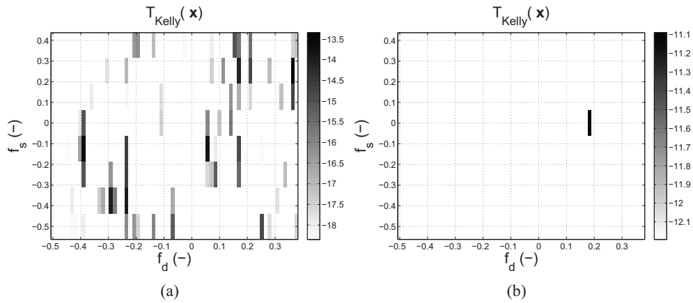
Figure 4. Statistique de test de Kelly pour la case distance numéro 256. (a) Données d'entraînement contenant les deux cellules contaminées 216 et 296. (b) Données d'entraînement contenant une seule cellule contaminée 296.
