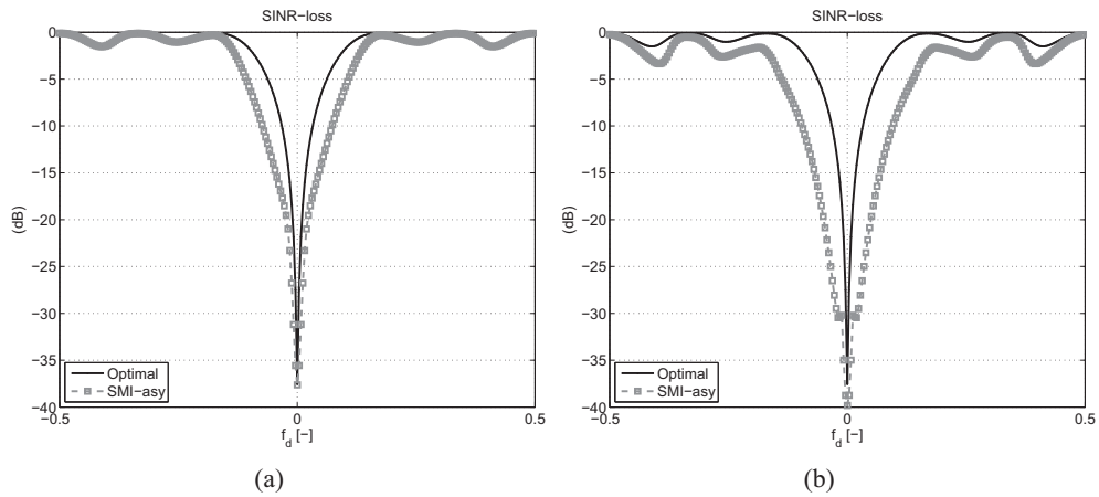
Figure 1. Pertes en SINR asymptotique dans un scénario avec transition brutale de la nature du fouillis. (a) Sur-estimation de l'étalement spectral, CNR_1 = CNR_2 = 24dB . (b) Sur-estimation de l'étalement spectral et de l'amplitude, CNR_1 = 24dB , CNR_2 = 40dB .
