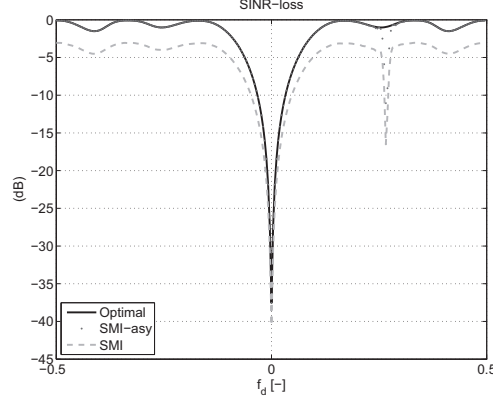
Figure 2. Pertes en SINR dans un scénario avec une cible secondaire dans l'intervalle d'entraînement.
