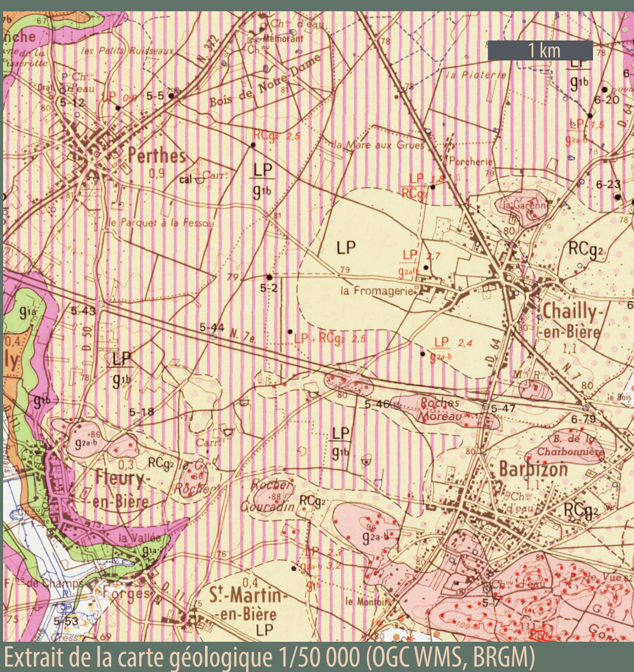
Extrait de la carte géologique 1/50 000 (OGC WMS, BRGM)
