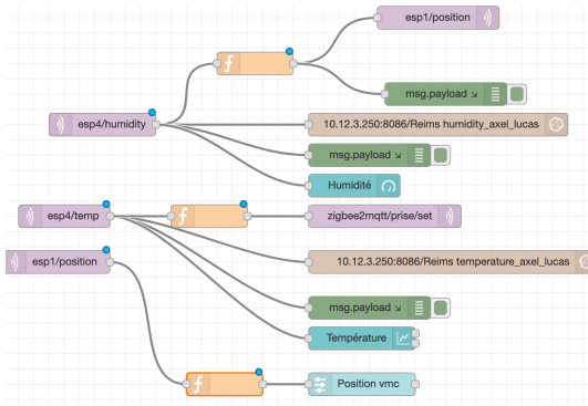
fig 2 : Exemple de programme Node-red
