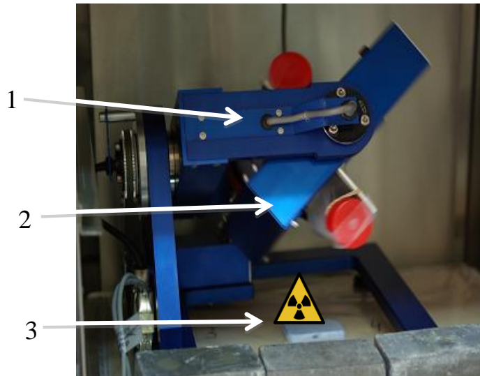
Fig.1. MARSimulateur combinant la simulation de la micropesanteur et le niveau de rayonnement présent à la SSI. 1) Random Positioning Machine (RPM) . 2) Plate forme tournante sur deux axes de rotation, qui peut porter des tubes et boîtes pétri . 3) Source de Nitrate de thorium dans un support cartonné scellé, et protégé par une barrière externe plastique . Le niveau de rayonnement au niveau du plateau est de 0.33 \pm 17 mSV/jour.
