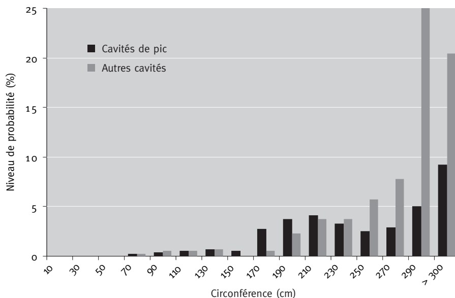
FIGURE 4 PROBABILITÉ DE DÉVELOPPEMENT DES CAVITÉS EN FONCTION DE LA TAILLE DE L'ARBRE (d'après Dufour, 2003 in Branquart et Liégeois, 2005)
