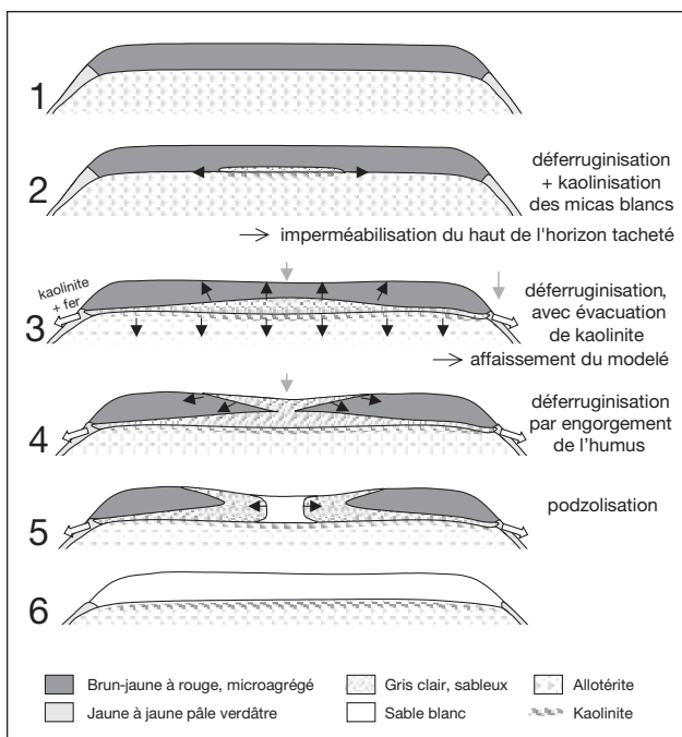
FIGURE 8 TRANSFORMATIONS D'UN PLATEAU SUR MIGMATITE PAR DÉFERRUGINISATION DUE À L'ENGORGEMENT HYDRIQUE, PUIS PAR PODZOLISATION
