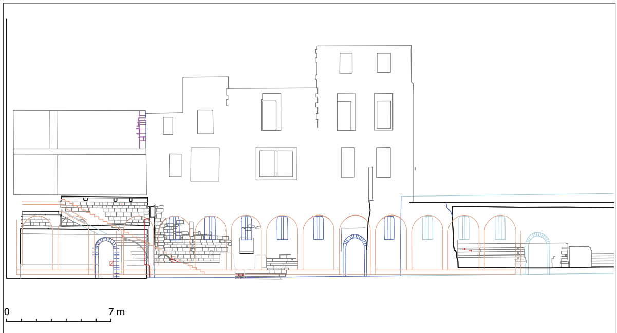
4 Ehemaliger Kreuzgang, tachymetergestütztes Teilaufmaß der Ostfassade des Westbaus mit Ansatz und Rekonstruktion einer geplanten Verlängerung der Westgaleriearkade nach Westen sowie der mutmaßlich Anfang des 13. Jahrhunderts eingebauten Treppenanlage (2014–2021).
