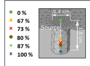
Figure 1 : Détail de l'électrode modélisé (modèle de la cellule conductive).
