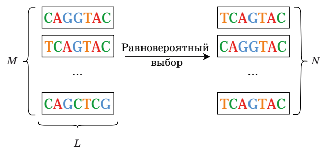
■ Рис. 3. Пример модели канала ДНК-памяти ■ Fig. 3. Example of DNA-storage channel model
