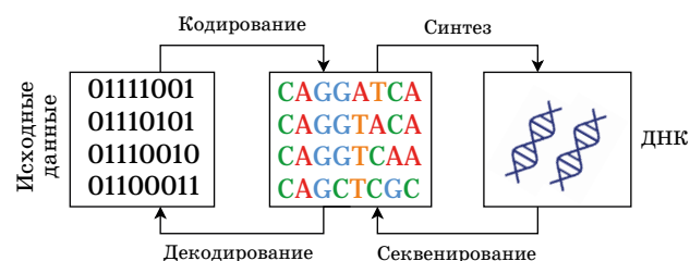
■ Рис. 1. Общая архитектура системы ДНК-памяти ■ Fig. 1. General architecture of DNA-based storage systems
