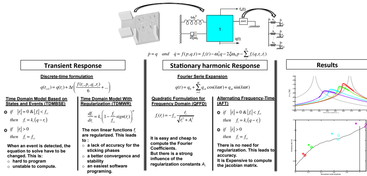
Figure 1: Différentes approches pour la simulation des réponses périodiques : - - - TDMWR; — QFFD; o-o-o AFT ; f_e = 4 ; f_e = 2 ; f_e = 0.5 ; f_e = 0.2 ; - · - Réponses linéaires dans le cas d'un système adhérent et d'un système glissant
