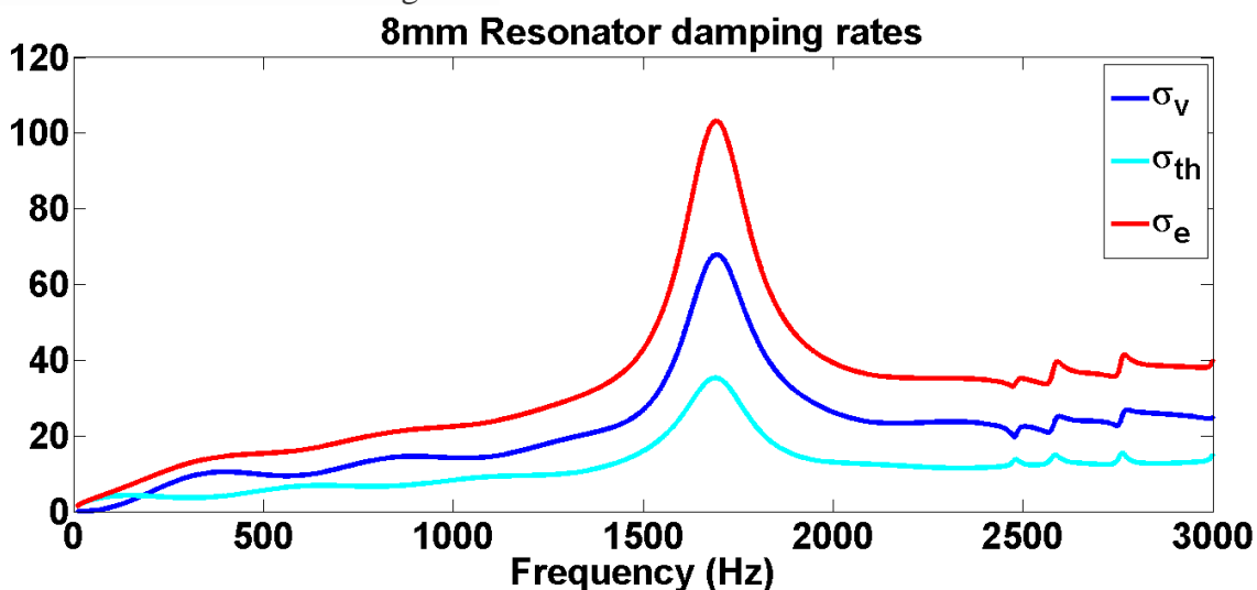
Figure 1 : taux d'amortissement : rouge) taux d'amortissement d'énergie, bleue) sa contribution visqueuse, cyan) sa contribution thermique.
