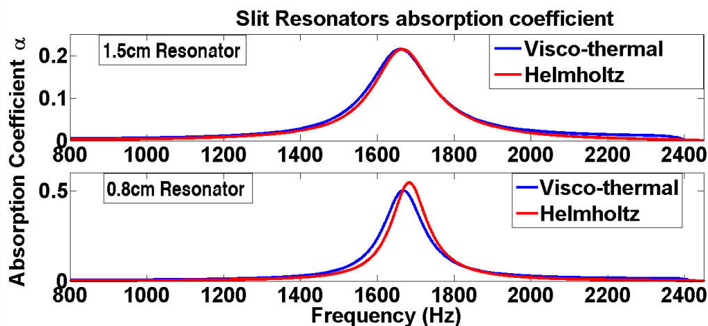
Figure 2: Coefficient d'absorption
