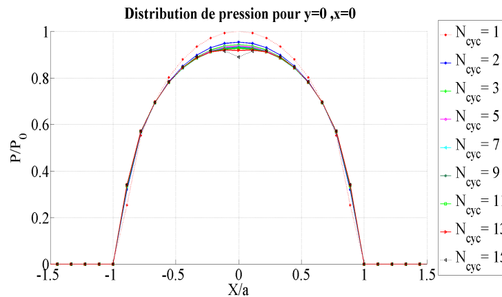
FIG. 4.3 – Evolution de la pression suivant la direction x en fonction du nombre de cycles
