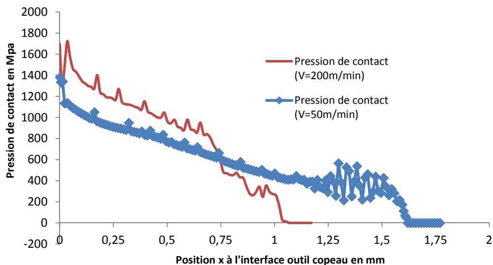
Figure 7. Evolution de la pression de contact à l'interface outil copeau
