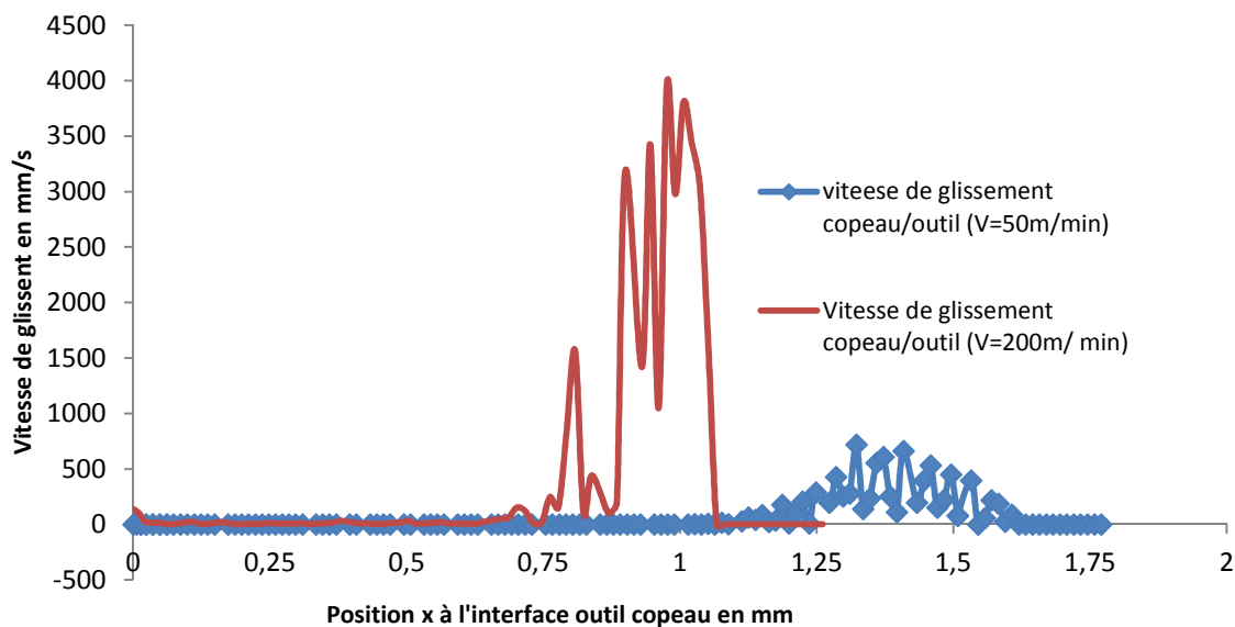
Figure 8. Evolution de la vitesse de glissement du copeau sur l'outil
