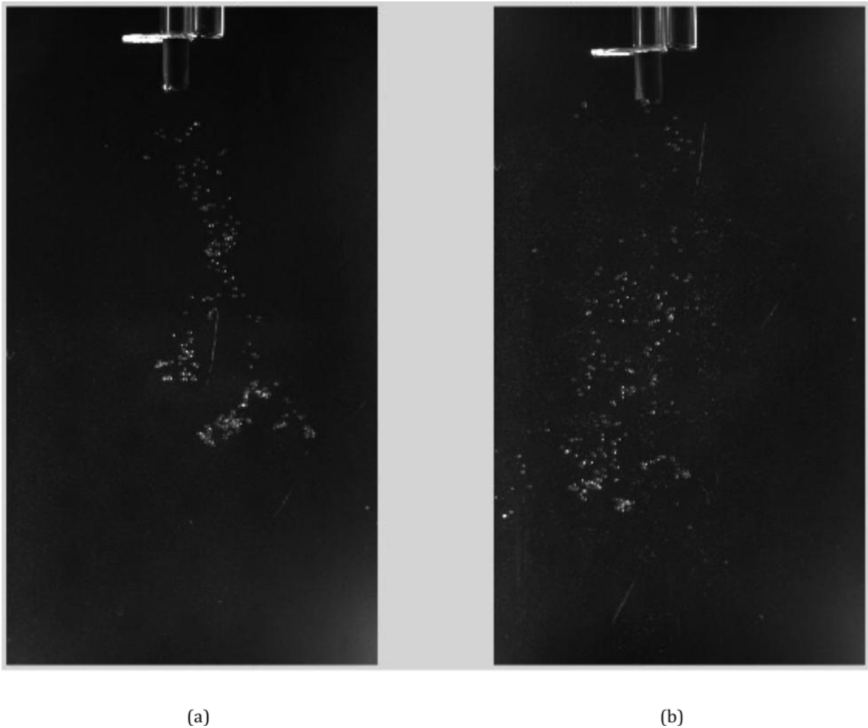
FIG. 7 – Sédimentation d'un nuage de particules (a) dans un fluide initialement au repos (b) à travers un réseau de tourbillons.
