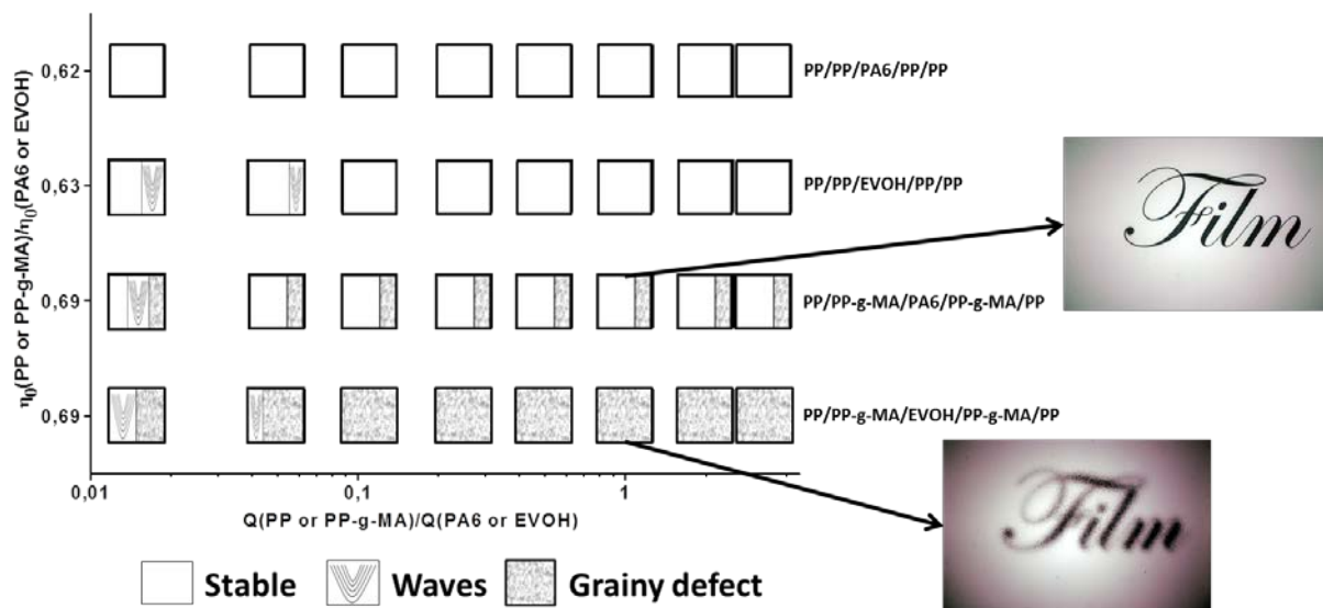
Fig. 2 Carte de stabilité à 230°C pour les films multicouches en fonction des ratios de débits (PP ou PP-g-AM)/(EVOH ou PA6)
