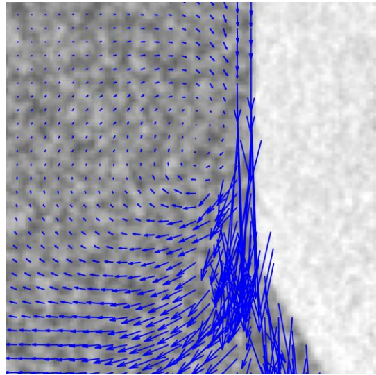
Figure 4- Vecteurs déplacement 2D autour du pieu après 2mm d'avancement de la tête du pieu continue. Les vecteurs sont amplifiés par un facteur 10 (Sable NE34).
