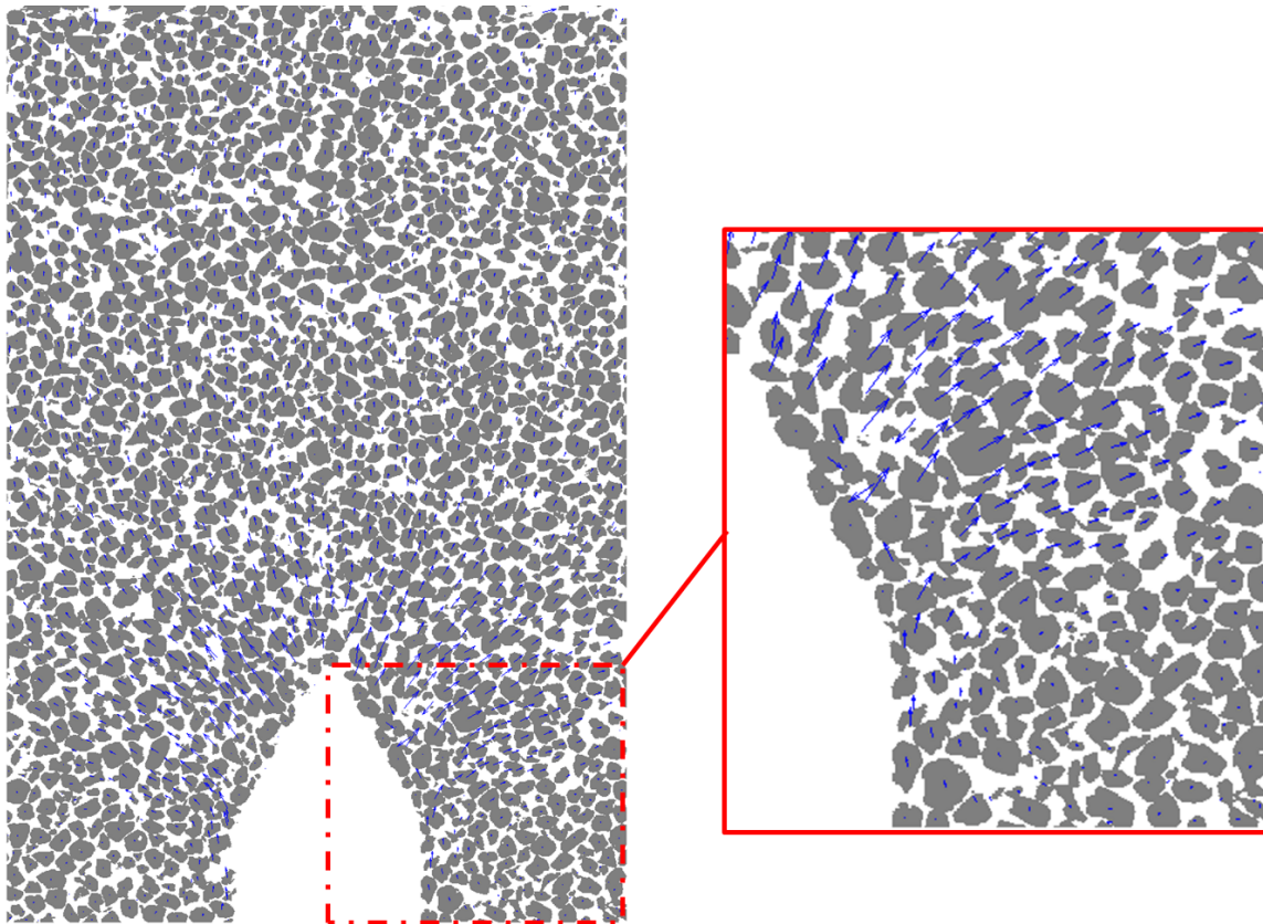
Figure 5- Vecteurs déplacement 2D autour du pieu après 2mm d'avancement de la tête du pieu discrète. Les vecteurs ne sont pas amplifiés (Hostun RF D_{50}=1,5\text{mm} )
