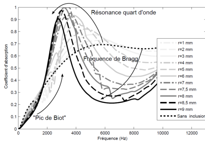
Figure 2 : coefficient d'absorption sous incidence normale pour un réseau périodique d'inclusions pleines en acier, de différents rayons.
