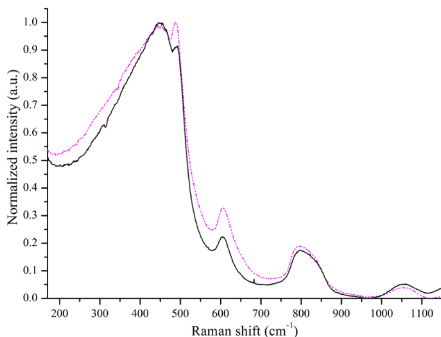
Figure 1: spectres Raman suite à une déformation plastique après compression hydrostatique (trait continu noir) et après la compression uniaxiale sur un micropilier (trait pointillé rose). Le taux de densification obtenue après déformation est de +4,6 % par rapport au verre initial « non densifié ».
