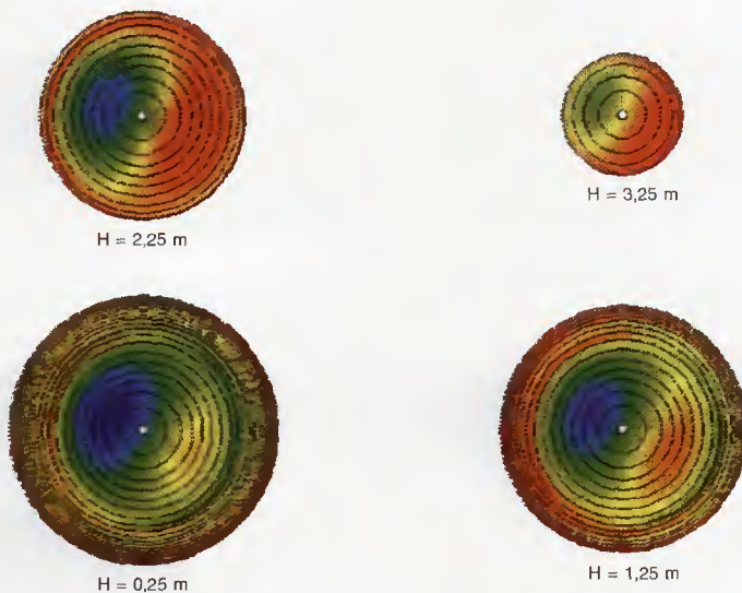
Figure 15 REPRÉSENTATION QUALITATIVE DES HÉTÉROGÉNÉITÉS DES CONTRAINTES LONGITUDINALES À DIFFÉRENTS NIVEAUX DU TRONC POUR UN PIN SIMULÉ À 20 ANS (d'après Fourcaud, 1995)
