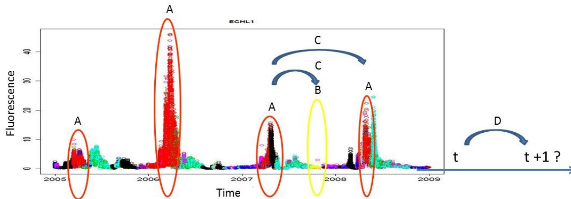
Figure 1. Évolution de la fluorescence mesurée par MAREL Carnot : identification des principaux états environnementaux et des éléments de dynamique à caractériser par classification et modélisation : (A) Événements courants, mais d'amplitude et de durée variables, (B) Événements rares, intermittents ou extrêmes, (C) dynamique entre les états et (D) prédiction des états.
