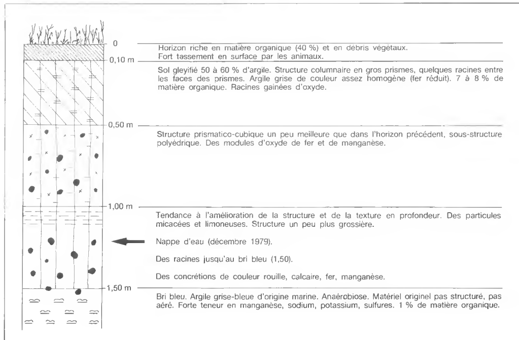
Figure 1 TRIAIZE : PROFIL PÉDOLOGIQUE
