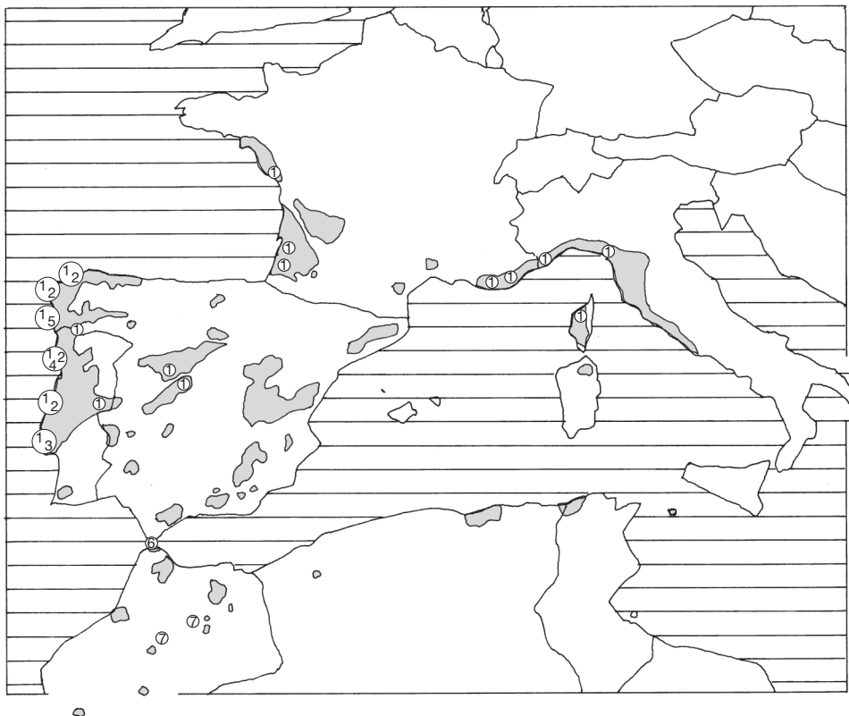
Figure 4 LOCALISATION DES DIFFÉRENTS MITOTYPES RÉVÉLÉS PAR L'ANALYSE PHYLOGÉOGRAPHIQUE de l'ADN mitochondrial des mâles de Matsucoccus feytaudi récoltés dans l'aire naturelle du Pin maritime
