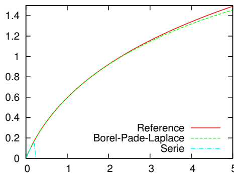
FIGURE 1 – Solutions approchées de l'équation d'Euler
