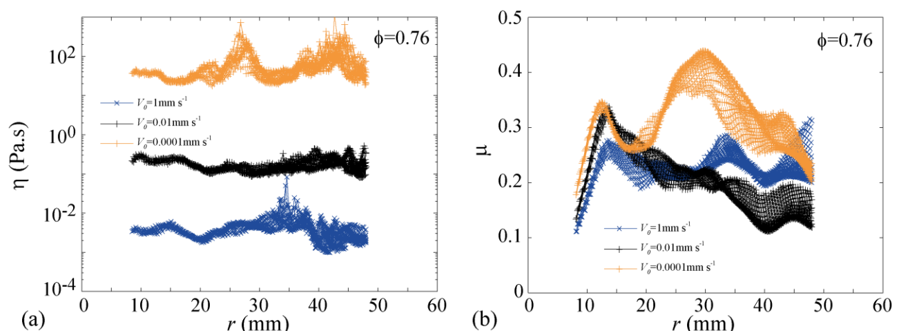
Fig. 5 – Evolution radiale suivant la direction \theta = 15^\circ \pm 5^\circ de la viscosité moyenne \eta (a) et du coefficient de friction moyen \mu (b) dans l'empilement de fraction volumique \phi = 0,76 autour de l'intrus pour différentes vitesses d'intrus V_0 = 10^{-4} (—+—), 10^{-2} (—+—), et 1 mm/s (—+—).
