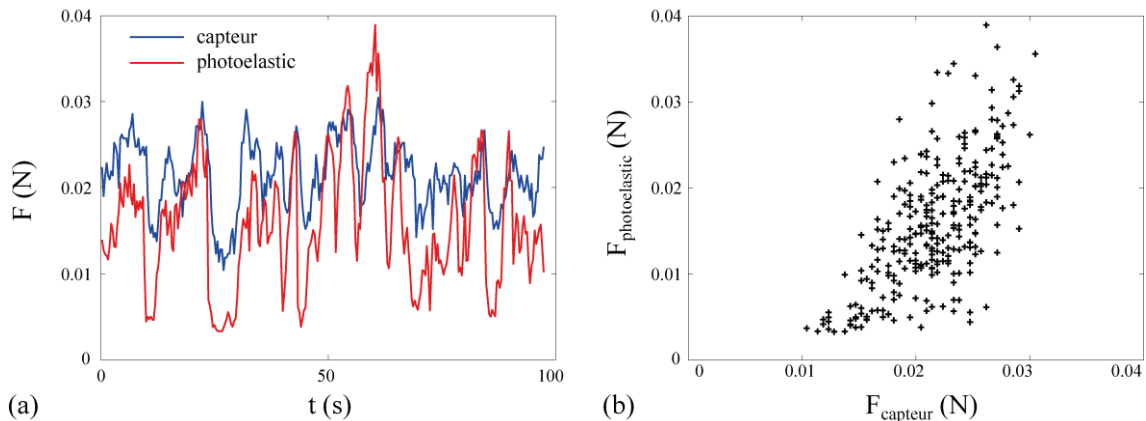
FIG. 2 – (a) Evolution temporelle de la force de traînée F sur le disque de diamètre 16 mm au cours de son mouvement à la vitesse V_0 = 0,1 mm/s : données du capteur piézoélectrique (—) et issues des analyses d'images polarisées (—). (b) Force de traînée instantanée déterminée par analyse d'images polarisées en fonction de la force mesurée par capteur piézoélectrique.
