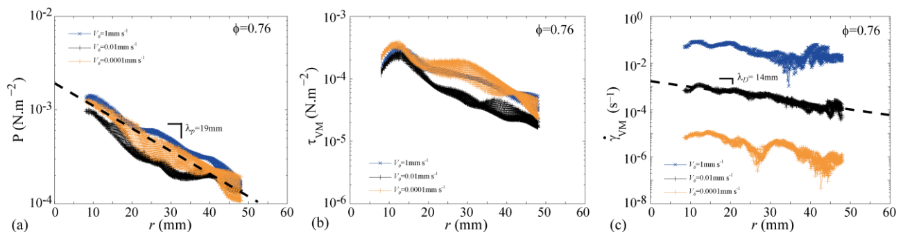
Fig. 4 – Evolution radiale suivant la direction \theta = 15^\circ \pm 5^\circ de la pression moyenne p (a), de la contrainte tangentielle moyenne \tau_{VM} (b) et du taux de déformation \dot{\gamma}_{VM} (c) dans l'empilement de fraction volumique \phi = 0,76 autour de l'intrus pour différentes vitesses d'intrus V_0 = 10^{-4} (—+—), 10^{-2} (—+—), et 1 mm/s (—+—).
