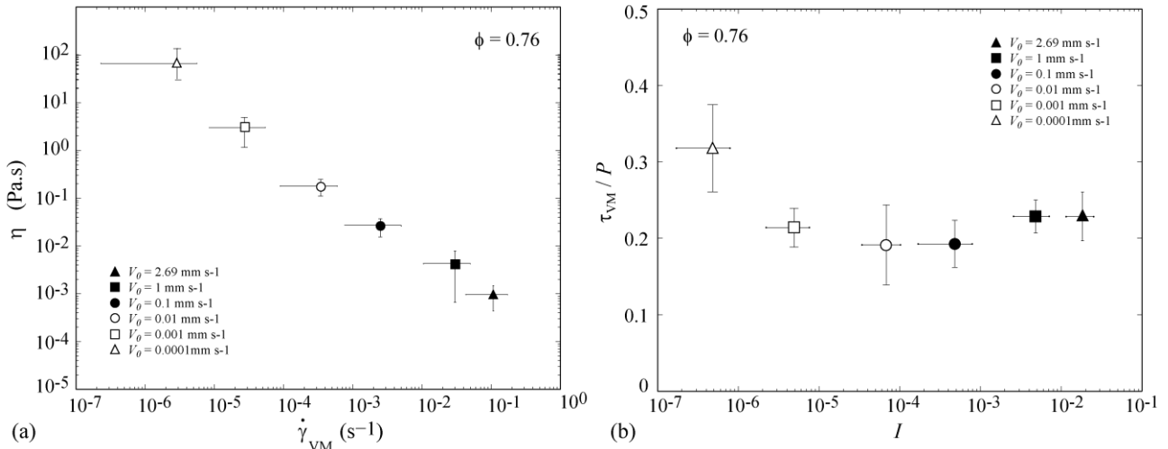
Fig. 6 – Evolution de la viscosité locale \eta en fonction du taux de déformation (a) et du coefficient de friction local \mu en fonction du nombre adimensionné local I (b) pour des expériences réalisées à différentes vitesses de traction 10^{-4} \leq V_0 < 3 mm/s dans un empilement de fraction volumique \phi = 0,76 .
