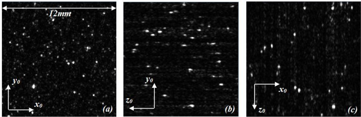
FIG. 4 – Coupes d'un volume reconstruit de 150 \times 150 \times 150 voxels 3 , plans x_0y_0 (a), y_0z_0 (b), x_0z_0 (c).
