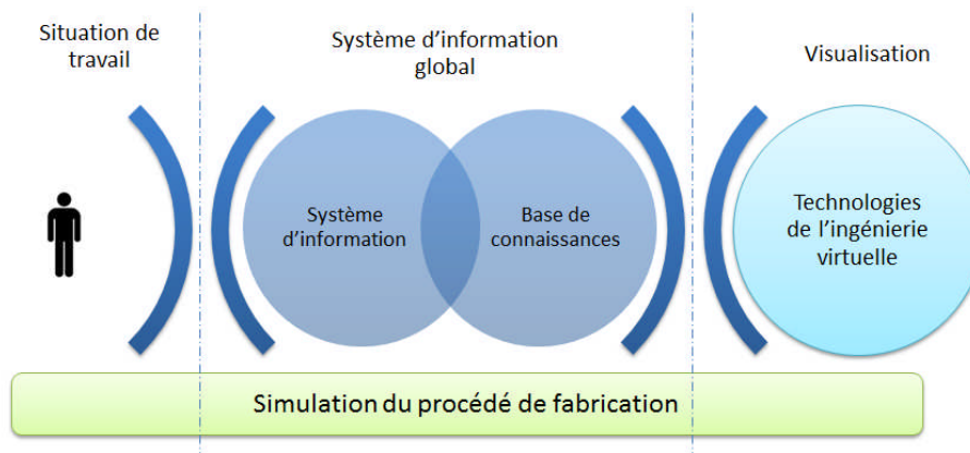
FIG. 3 – Architecture globale du système envisagé
