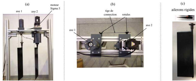
FIGURE 2 – Photographies du système d'oscillation à double ailerons : vue aval (a), vue de dessus (b) et aileron rigide (c).
