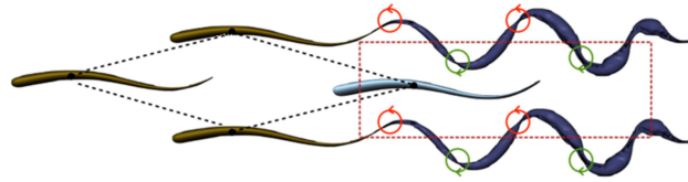
FIGURE 1 – Illustration de la nage en groupe comme décrite par [2]. Le losange pointillé montre la formation en losange et le rectangle en pointillé montre l'allée BvK obtenue entre deux sillages de BvK inversés.
