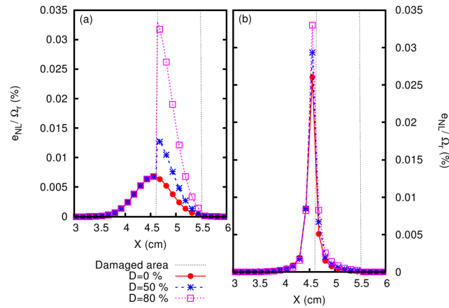
FIGURE 4 – Contribution non-locale près d'une zone endommagée : (a) formulation originale ; (b) formulation basée sur les interactions.
