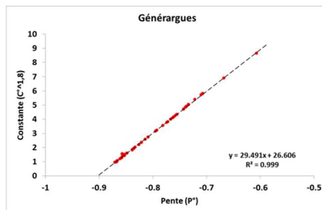
Fig. 2 Relation entre l'exposant P^\circ du modèle de puissance et la constante C^\circ du même modèle pour la station de Générargues (Gardon)
