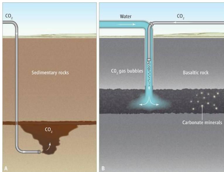
Figure 1 : Les deux approches actuelles pour le stockage géologique du CO 2 : a) stockage dans des formations sédimentaires : le CO 2 est injecté sous forme supercritique et piégé par une roche de couverture imperméable ; b) la méthode CarbFix : le CO 2 est dissout dans de l'eau concomitamment à son injection dans un réservoir basaltique où il réagit avec la roche hôte pour former des carbonates – Illustration reproduite avec la permission de Matter et al. , 2016.
