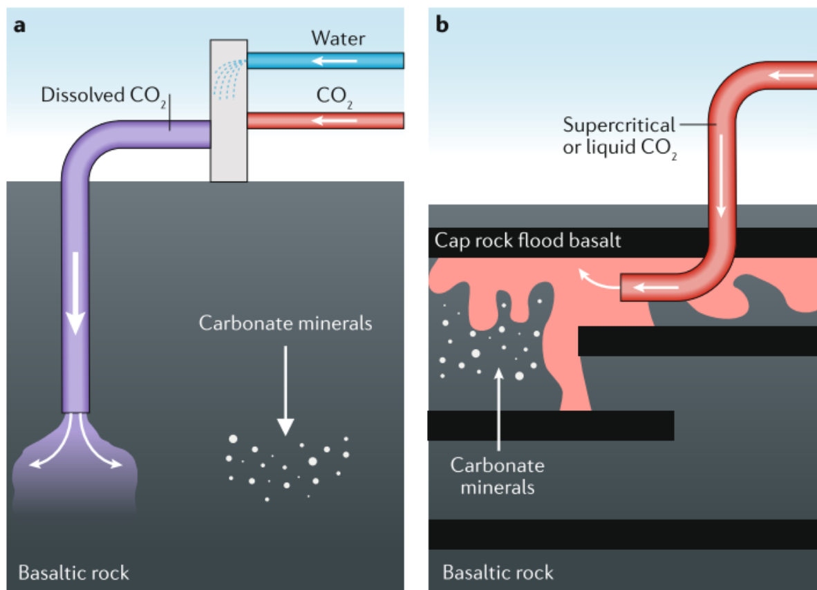
Figure 3 : Résumé des deux projets pilotes de minéralisation in-situ : a) dans le projet CarbFix, le CO 2 arrive dans le réservoir complètement dissout ; b) dans le projet Wallula, le CO 2 est injecté sous forme supercritique (illustration reproduite avec la permission de Snæbjörnsdóttir et al. , 2020).
