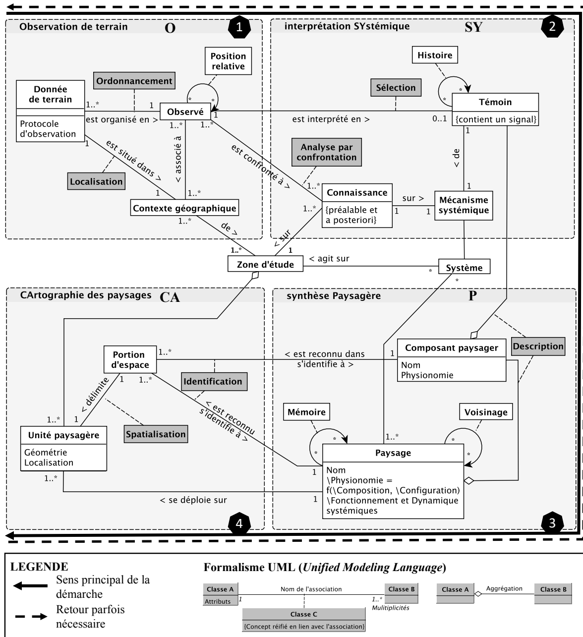
Figure 2 : La méthode OSYPCA d'analyse paysagère.
