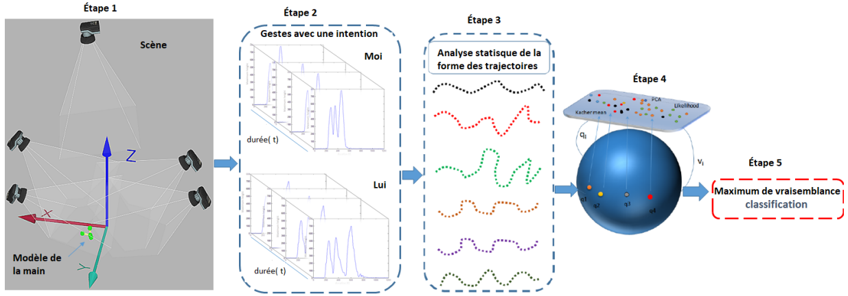
FIGURE 1 – Vue générale de la méthode proposée.
