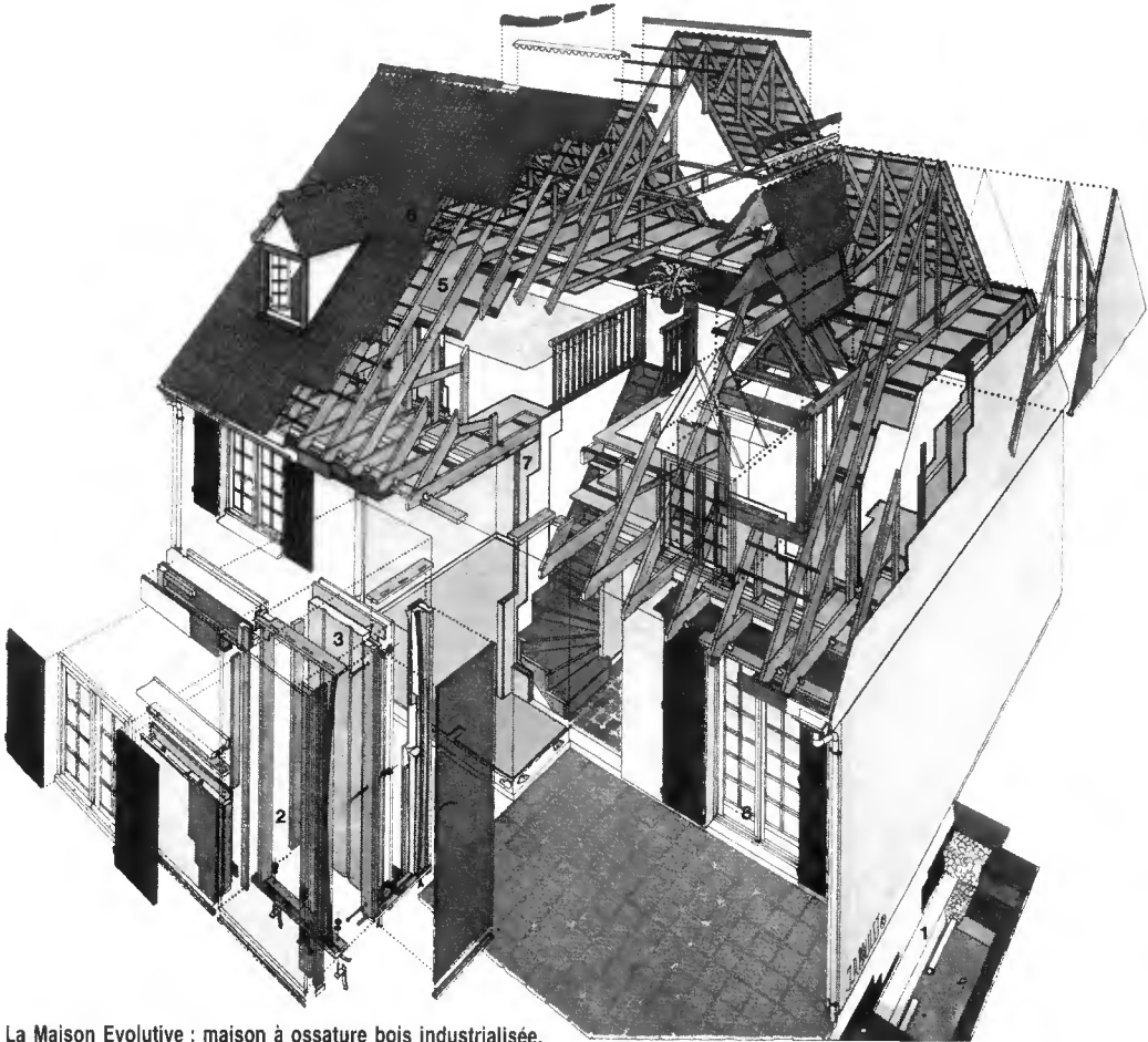
La Maison Evolutive : maison à ossature bois industrialisée.
