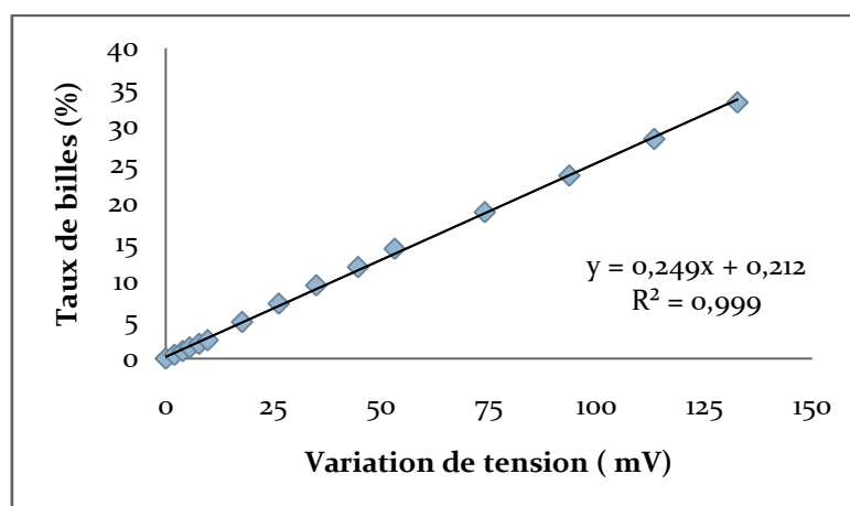
FIG. 3 – Evolution du taux de billes de verre en fonction de la tension.
