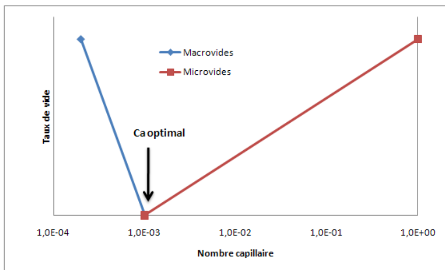
FIG. 2 – Taux de vides en fonction du nombre capillaire
