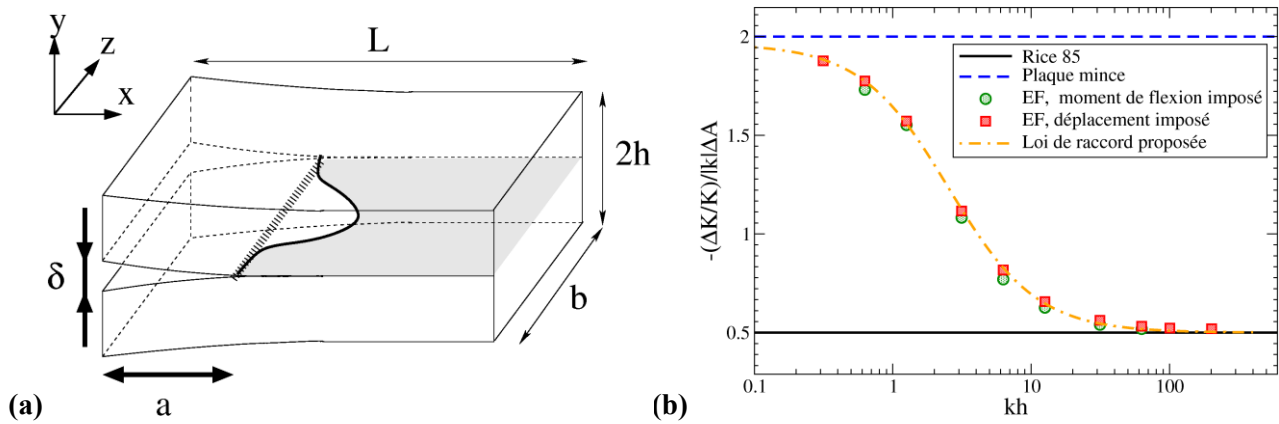
FIG. 1 – (a) Schéma d'un essai de clivage représentant une fissure plane dans une éprouvette de taille finie. (b) Amplitude normalisée du taux de restitution d'énergie pour une perturbation sinusoïdale du front de fissure en fonction de la fréquence de la perturbation.
