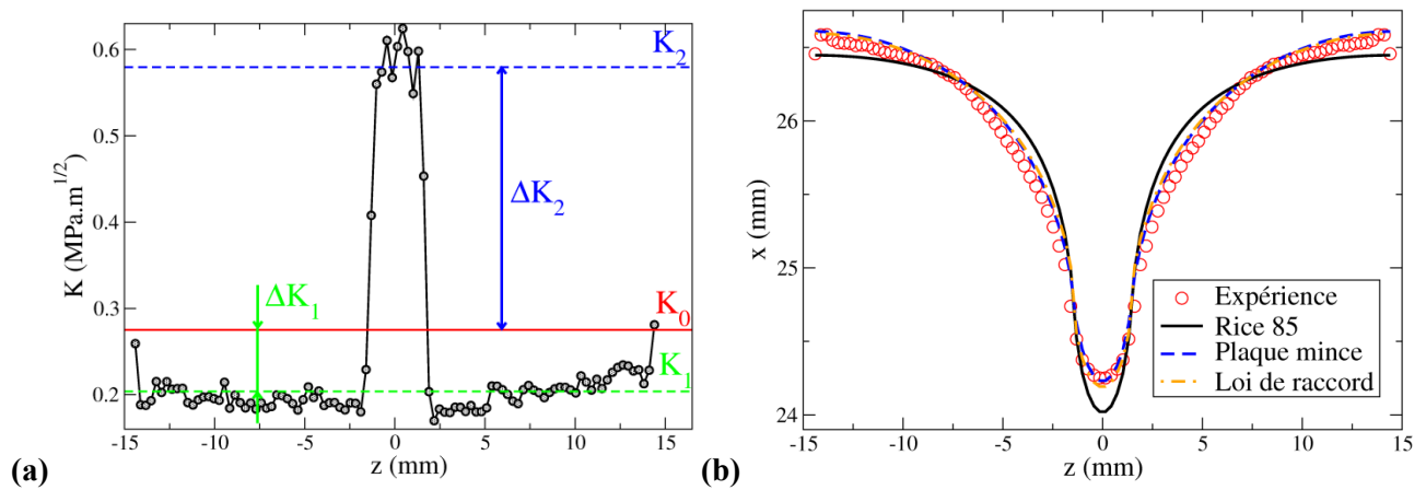
FIG. 3 – (a) Taux de restitution d'énergie calculé par la méthode des éléments finis en fonction de la position longitudinale le long du front de fissure. (b) Position de la fissure. Les données expérimentales corrigées (cercles) sont comparées aux différents modèles de ligne élastique (courbes continues et discontinues).
