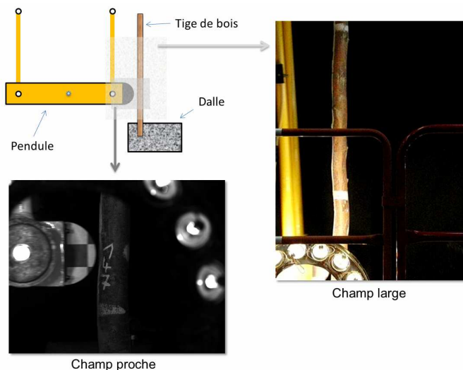
FIG. 2 – Schéma du pendule de Mouton-Charpy utilisé et champs de prise de vue associés aux caméras rapides. Un champ proche pour caractériser l'interaction bloc/arbre et un champ large pour mesurer la cinématique globale de la tige.
