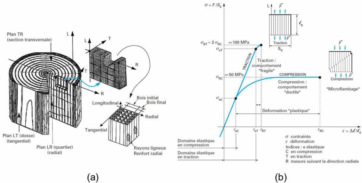
FIG. 1 – Description structurale du bois à l'échelle de la section (a) Exemple qualitatif du comportement mécanique en traction et compression (b) [8].
