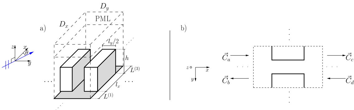
FIGURE 2 – a) cellule élémentaire du réseau periodique infini en x et y . b) ondes entrantes et sortantes de chaque côté de la cellule élémentaire, vue du dessus.
