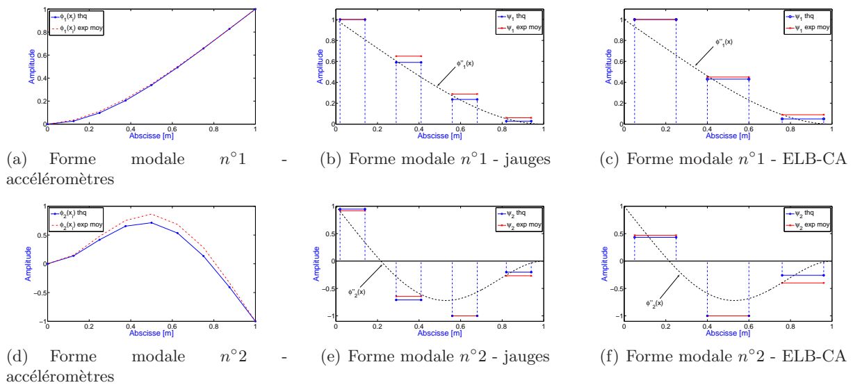
FIGURE 4 – Formes modales obtenues avec la TOC à partir des signaux des accéléromètres, des jauges et des ELB-CA.
