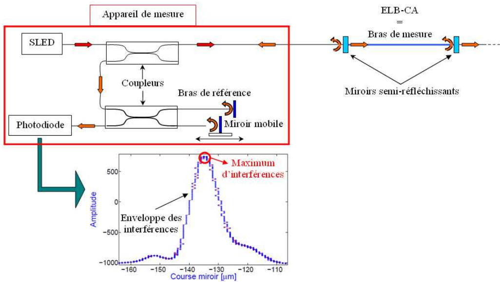
FIGURE 1 – Schéma de principe de l'interrogateur optique.
