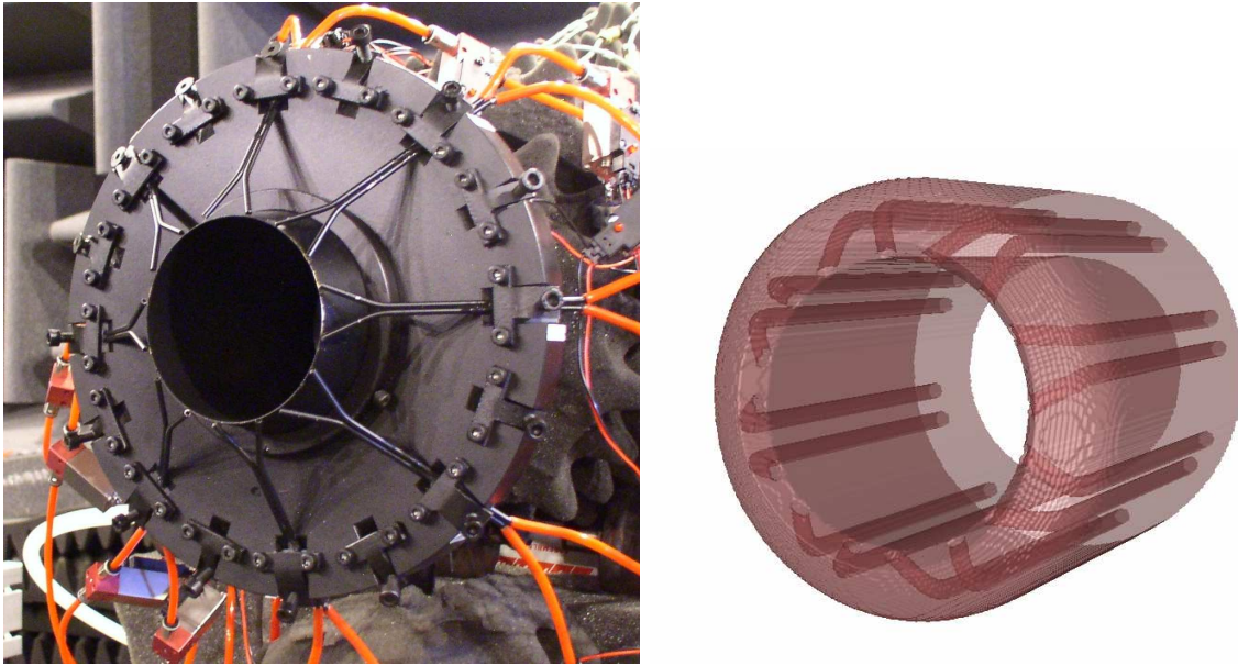
FIG. 1 – Gauche : dispositif expérimental de fluidevrons [6]. Droite : vue de la géométrie modélisée par frontières immergées.
