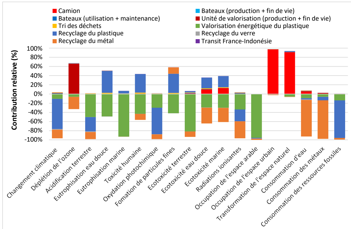
Figure 5 : Résultats de l'analyse de cycle de vie du schéma d'économie circulaire sur 20 ans
