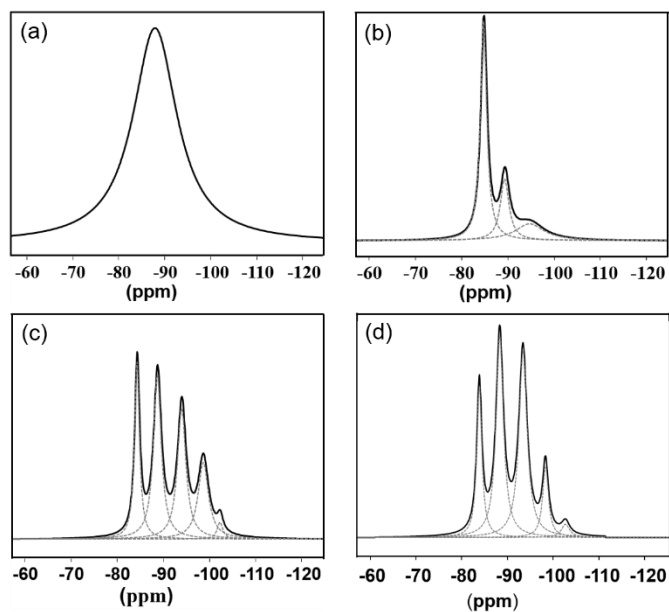
Fig. 7 ^{29}\text{Si} NMR spectra of amorphous precursor (a), FAU-1- nano (b), FAU-2- nano (c) and FAU-3- micron (d).
